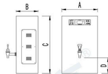
HZK-20A A: 355 B: 217 C: 566 D: 165
