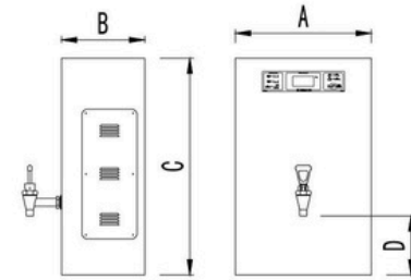
HZK-30A A: 405 B: 247 C: 616 D: 165
