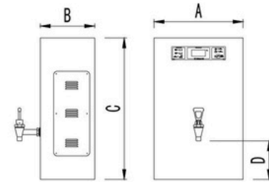
HZK-10A A: 305 B: 187 C: 466 D: 165
