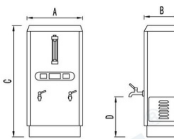
ZK-15K A: 556 B: 335 C: 1060 D: 250
