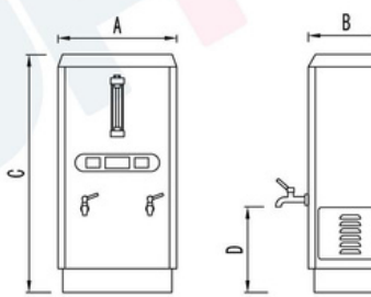
ZK-6K A: 401 B: 257 C: 804 D: 260
