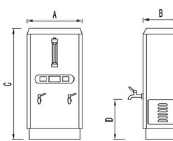
ZK-12K A: 450 B: 277 C: 980 D: 260
