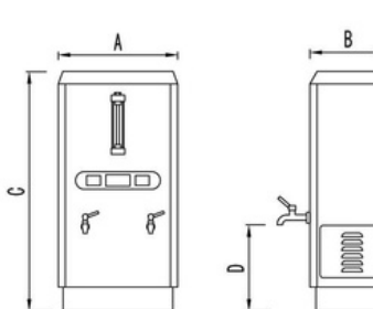
ZK-9K A: 446 B: 277 C: 880 D: 260
