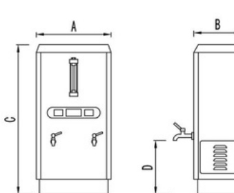
ZK-18K A: 556 B: 335 C: 1160 D: 250
