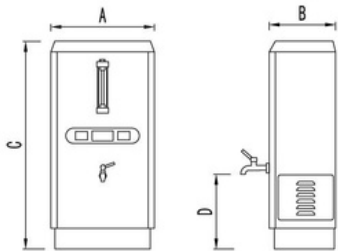
ZK-3K A: 401 B: 257 C: 704 D: 210
